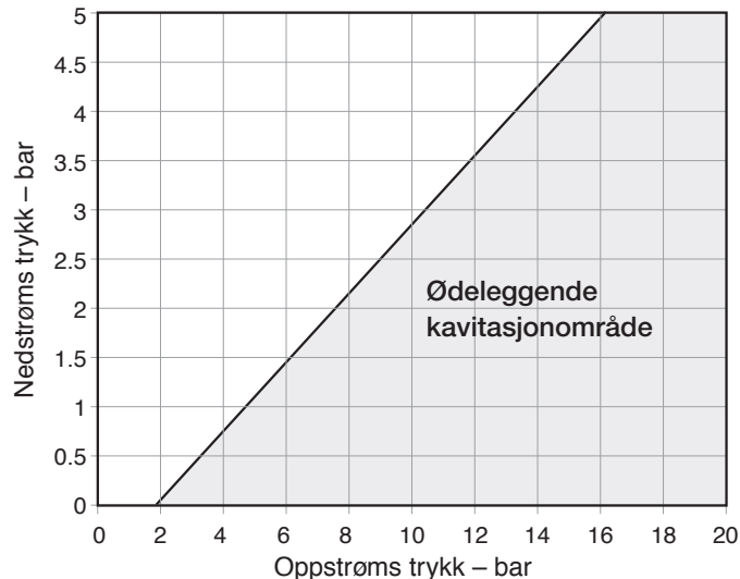
700-EN, 700, 800
